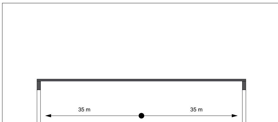
Fluchtweglänge bei zwei oder mehreren Ausgängen
