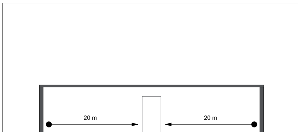
Fluchtweglänge bei einem Ausgang
