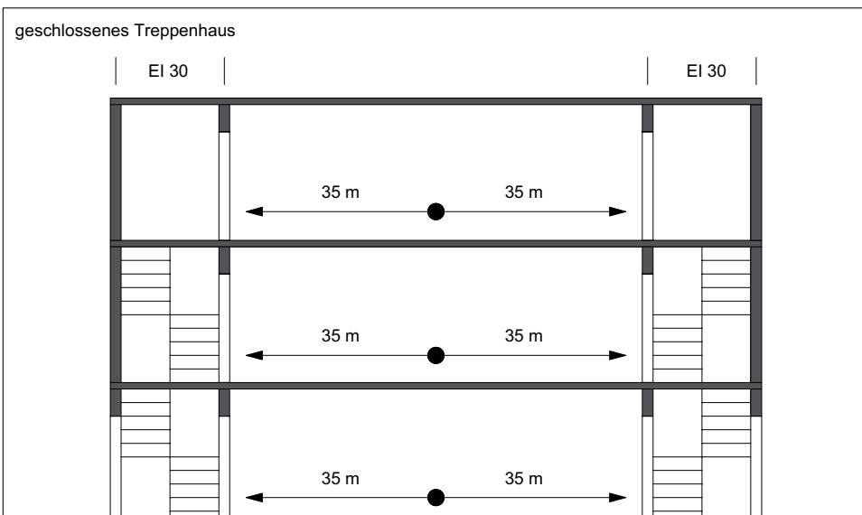
Fluchtweglänge bei zwei oder mehreren, geschlossenen Treppenhäusern (EI 30)
