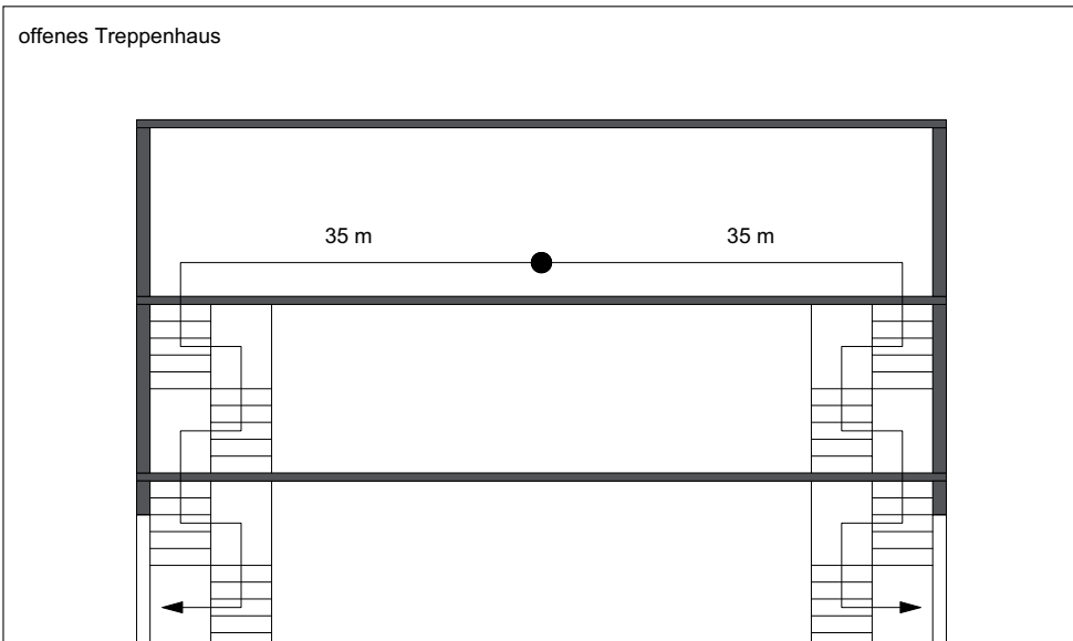
Fluchtweglänge bei zwei oder mehreren, offenen Treppenhäusern
